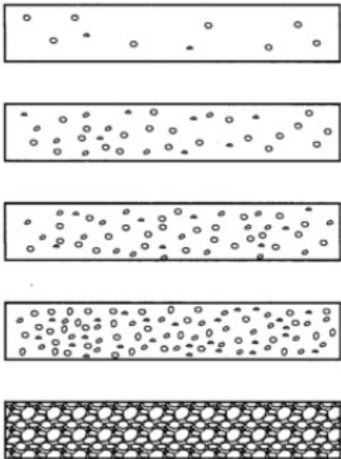
图 F.1 涂层黏结面孔隙率等级
