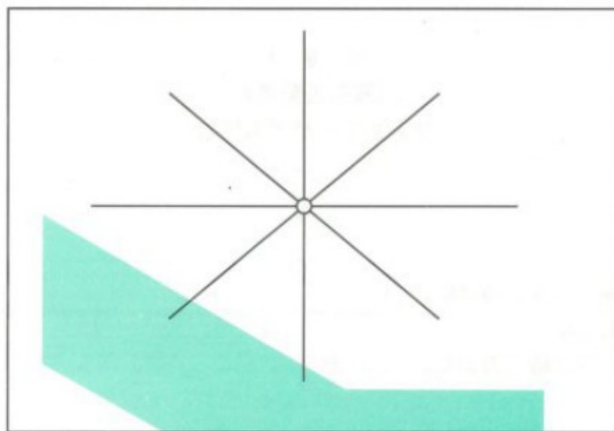
图 C.1 在试件上划透涂层的放射线
