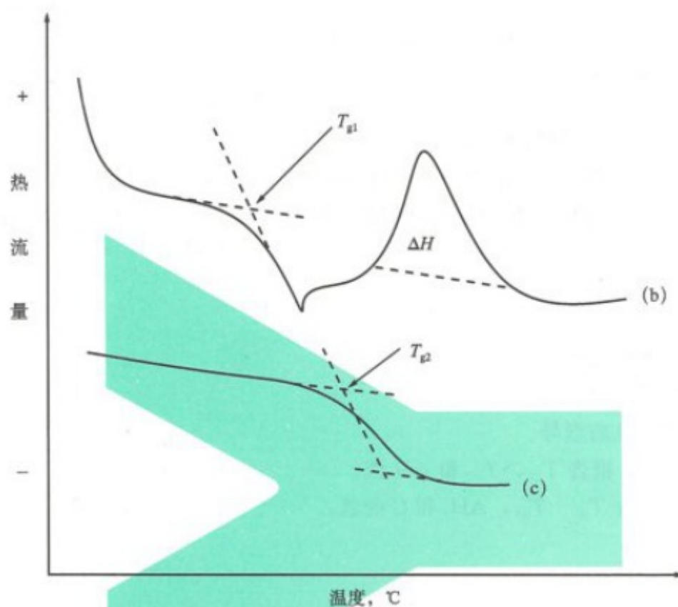
图 B.1 对环氧粉末热扫描
