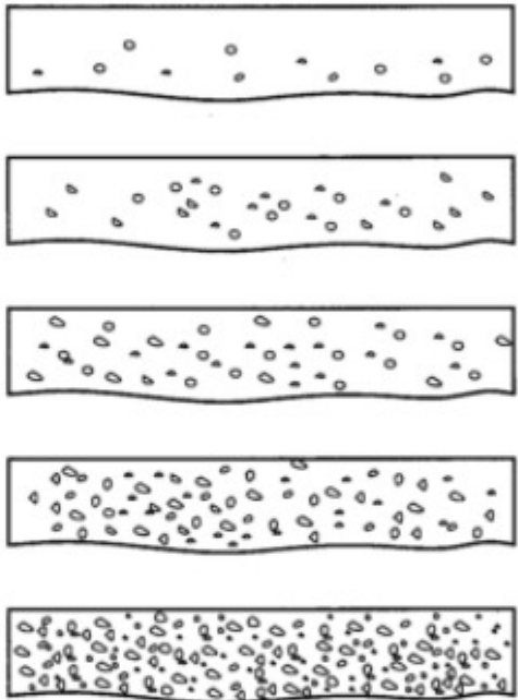
图 F.2 涂层断面孔隙率等级
