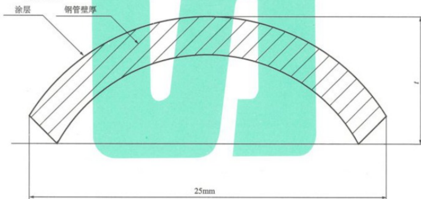
图 D.1 抗弯曲试验试件厚度的确定
