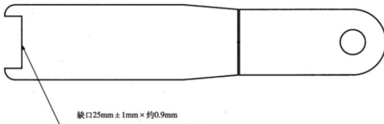
图 A.1 拉延板
