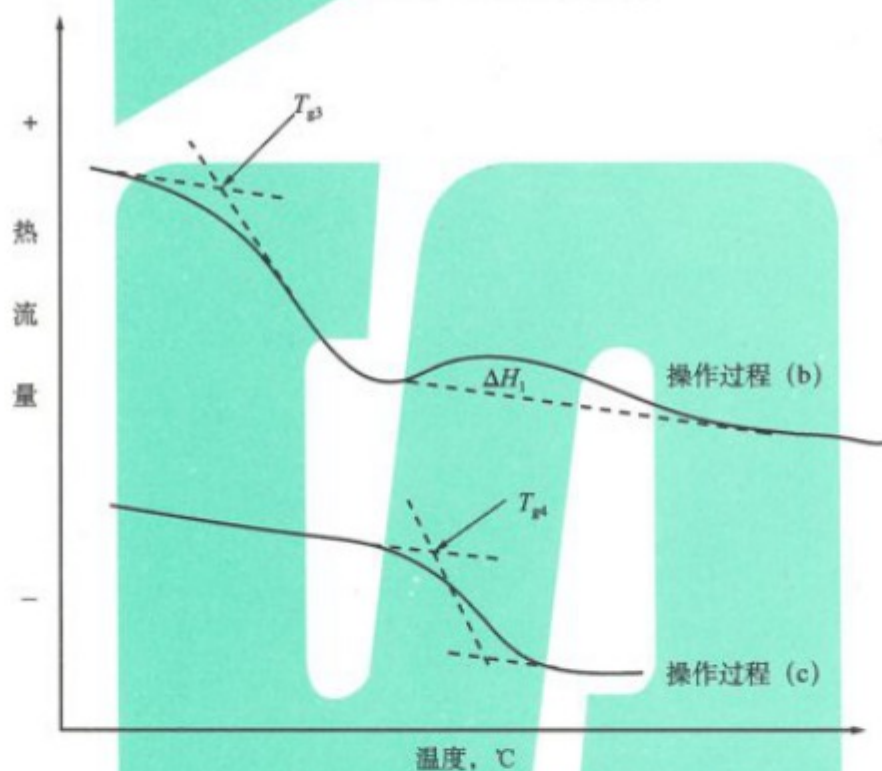
图 B.2 对涂层热扫描
